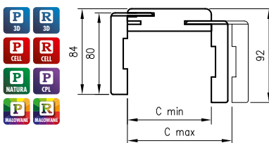
Prierez TUN zo zásuvnou časťou N63
