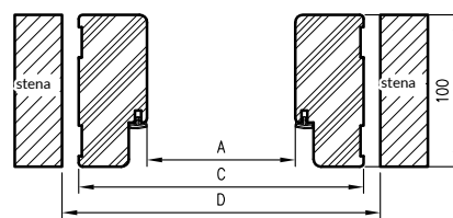
pre poldrážkové dvere jednokrídlové
