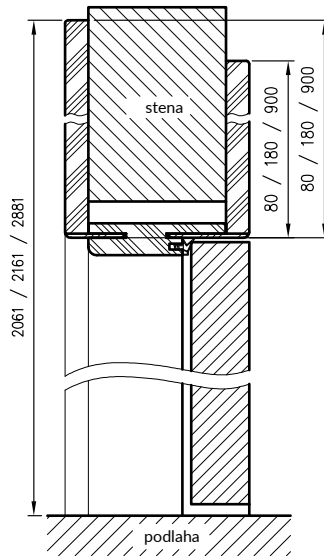
Zvislý prierez ORB Maľovaná, spojenie 0°
