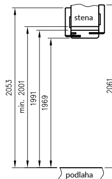
Prierez TUN zo zásuvnou časťou T80
