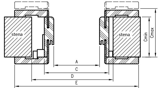
Pozdĺžny prierez ORB
