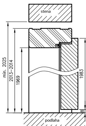
Zvislý prierez OP pre poldrážkové dvere
