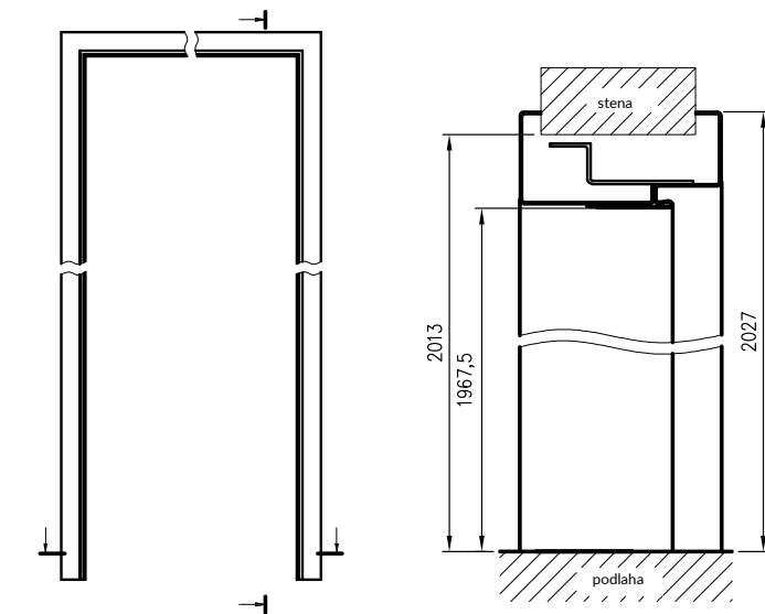
Varianty zárubní podľa hrúbky steny
