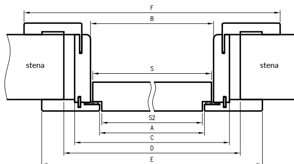
Pozdĺžny prierez ORO
