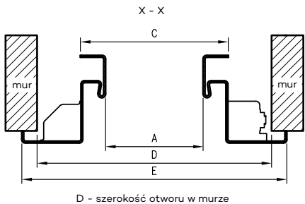
D – szerokość otworu w murze
