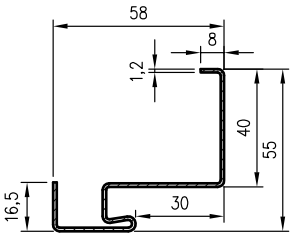
Profil ościeznicy OSMK
