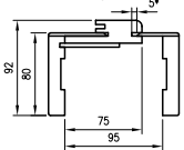
Przekrój ORB 075
