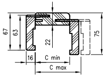
Przekrój TUN z kąt. T63
