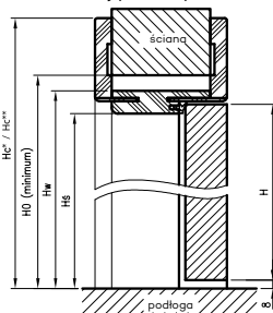
Przekrój pionowy ORB
