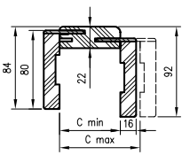
Przekrój TUN z kąt. T63
