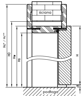
Przekrój pionowy OR
