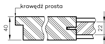
Przekrój poziomy drzwi Elsa
