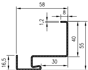
Profil ościeznicy OSMK
