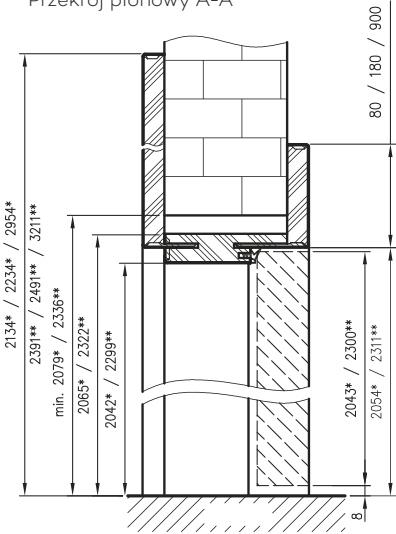
Przekrój pionowy A-A
