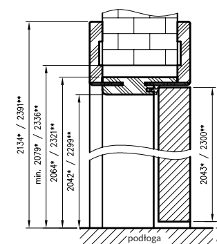
przekrój pionowy
