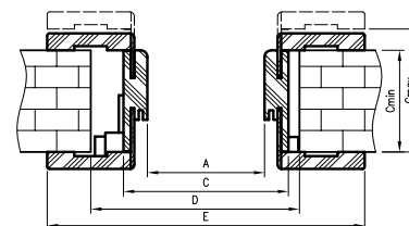
przekrój poziomy
