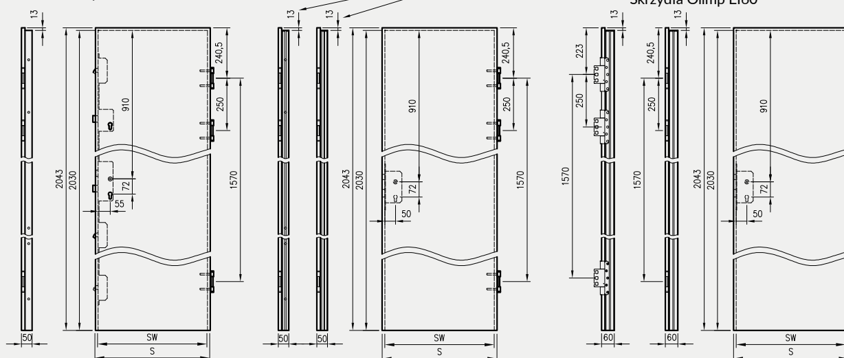
Skrzydła Olimp EI60**
