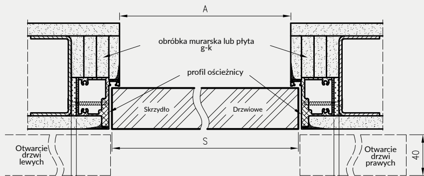
Przekrój poprzeczny dla drzwi Sara Eco2 bezprzylgowe - otwierane na zewnątrz
