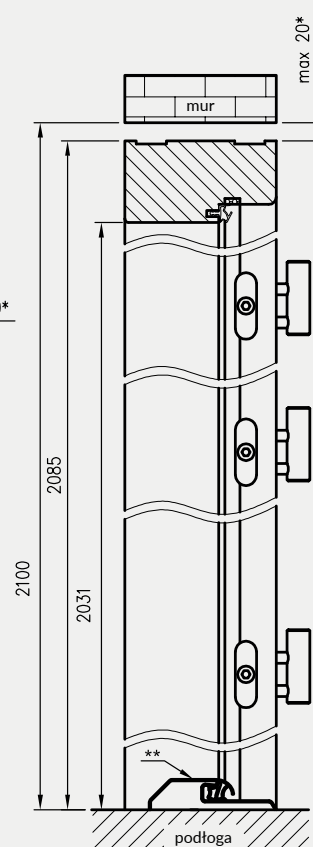
Przekrój pionowy OD ATHOS
