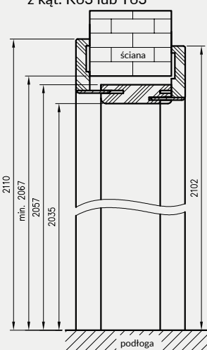
Przekrój pionowy tunelu regulowanego z ką. K63 lub T63
