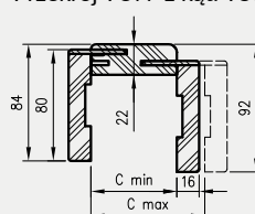
Przekrój TUN z ką. T63
