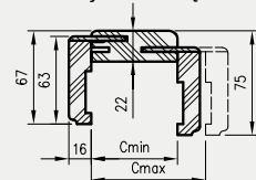
Przekrój TUN z ką. K63
