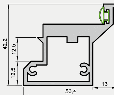
Profil ościeżnicy z uszczelką
