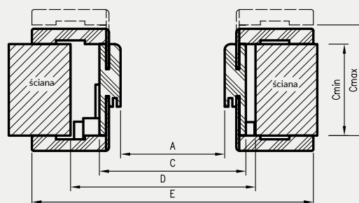
Przekrój poziomy ORB
