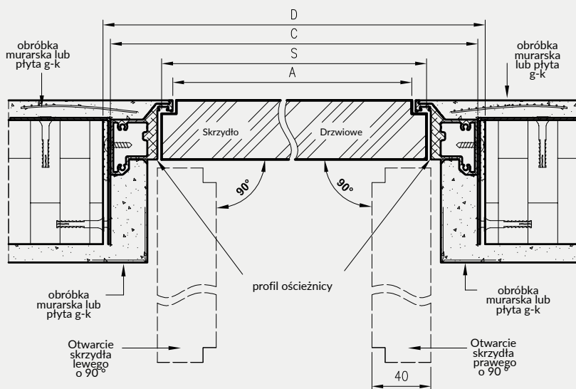
Przekrój poprzeczny dla drzwi Sara Eco2 przylgowe - otwierane do wewnątrz
