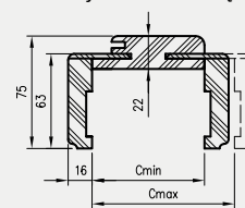
Przekrój OR/ORC z ką. K63
