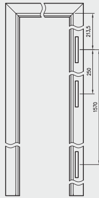
metal door frame for hinges VX 7939
