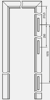
metal door frame for hinges VX 7939
