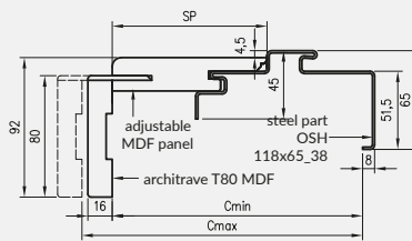
door frame profile
