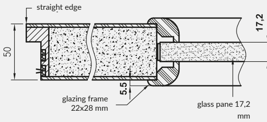
Fire resistant door leaf Olimp EI30
