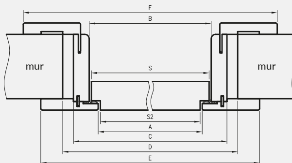
Przekrój poziomy ORO
