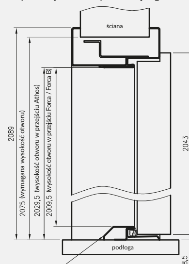
Próg stały (stalowy) do drzwi Forca i Forca B lub uszczelka opadająca w drzwiach Athos
