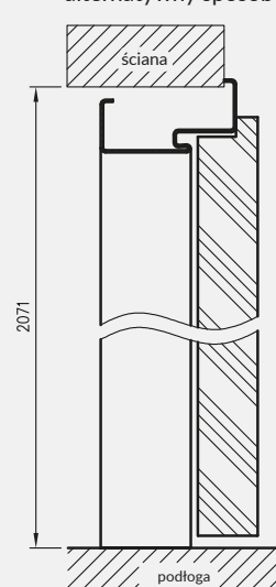
przekrój pionowy alternatywny sposób montażu
