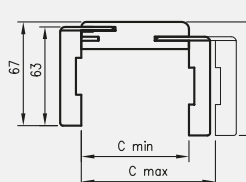
Przekrój TUN z ką. T63
