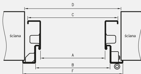
przekrój poziomy ościeznicy w murze
