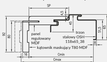
profil ościeznicy
