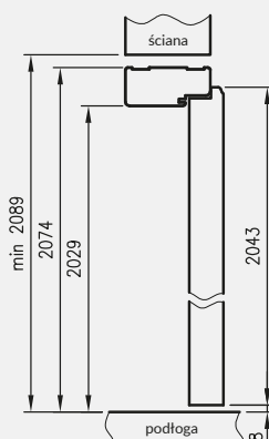
Przekrój pionowy drzwi przylgowych
