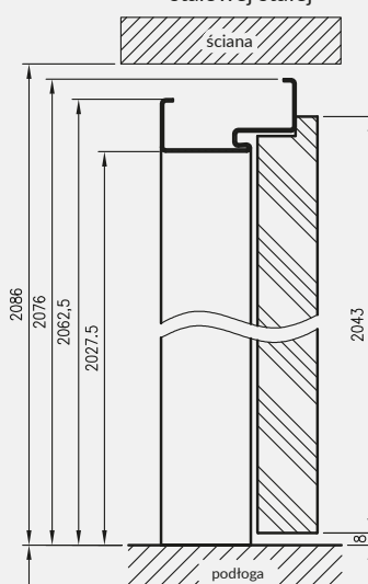
przekrój poprzeczny alternatywny sposób montażu
