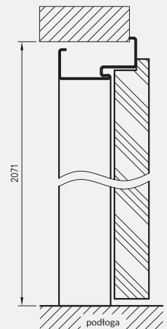
Przekrój pionowy alternatywny sposób montażu
