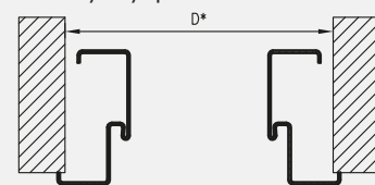
przekrój poprzeczny alternatywny sposób montażu
