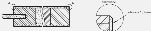
Przekrój ramia skrzydła bezprzylgowego
