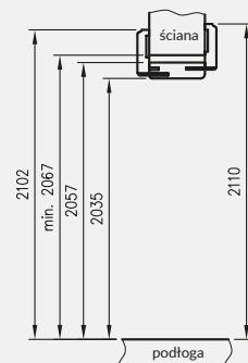
Przekrój pionowy tunelu regulowanego z ką. T80
