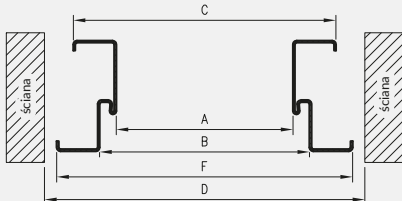
Przekrój poprzeczny
