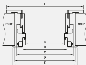
przekrój poziomy ościeznicy w murze
