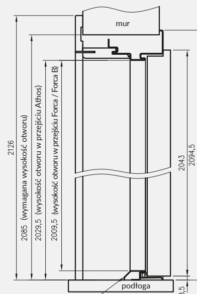
przekrój pionowy
