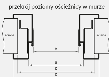
przekrój poziomy ościeżnicy w murze
