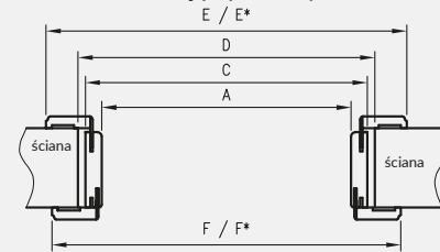
Przekrój poprzeczny TUN
