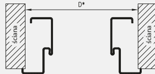
Przekrój poprzeczny alternatywny sposób montażu
