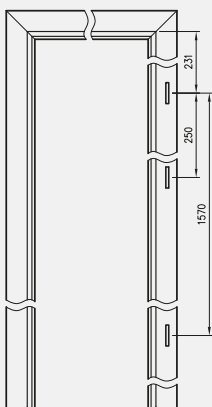
Przekrój ościeznicy metalowej do drzwi Olimp
