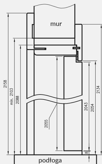
Przekrój pionowy ORO
