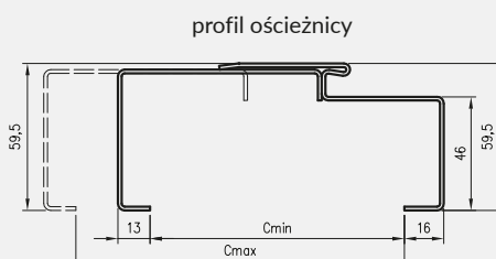
profil ościeżnicy
