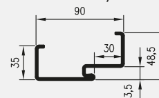
Profil ościeżnicy stalowej
