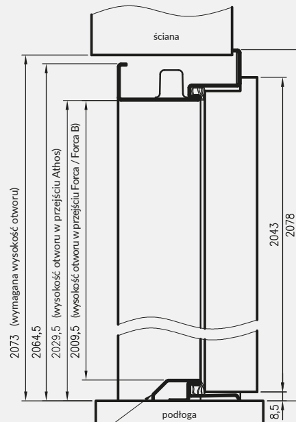
przekrój pionowy
