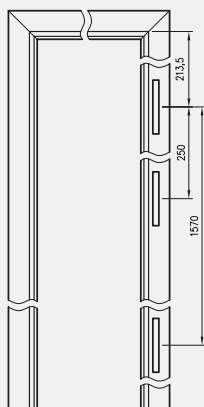
ościeżnica metalowa pod zawiasy VX 7939
