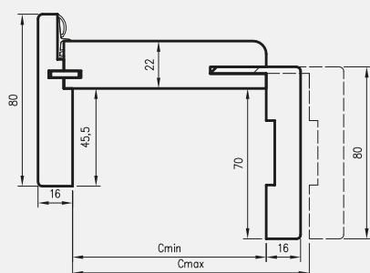
Profil ościeżnicy
