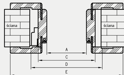
Przekrój poziomy OR
