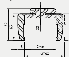
Przekrój OR/ORC Natura z kąt. N63
