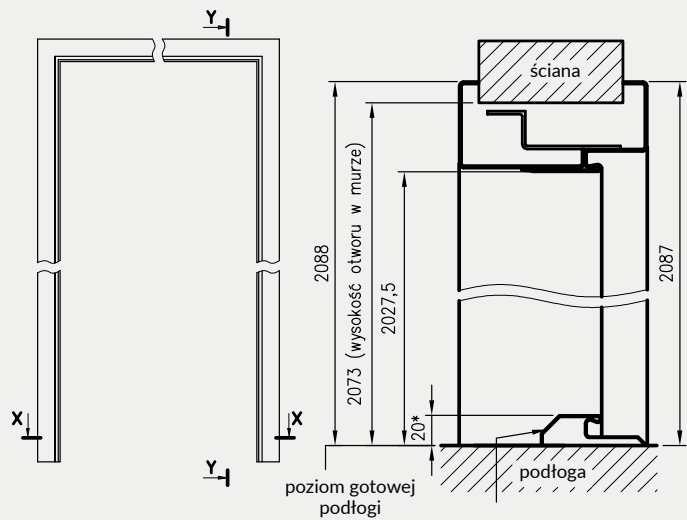
Profil ościeżnicy OSR z kątownikiem domykającym T57
