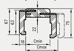
Przekrój TUN Natura z ką. N63
