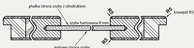
Przekrój poziomy drzwi VETRO B5, B10-B11
