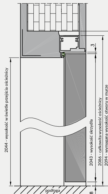
Przekrój pionowy drzwi Sara Eco
