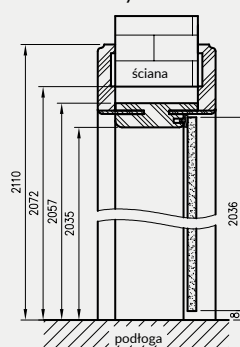
Przekrój pionowy drzwi szklanych ORC
