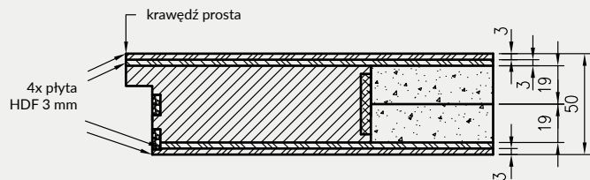
Skrzydło drzwiowe przeciwpożarowe Athos EI30
