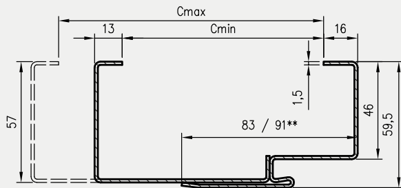
Profil ościeżnicy OSR z kątownikiem domykającym T57
