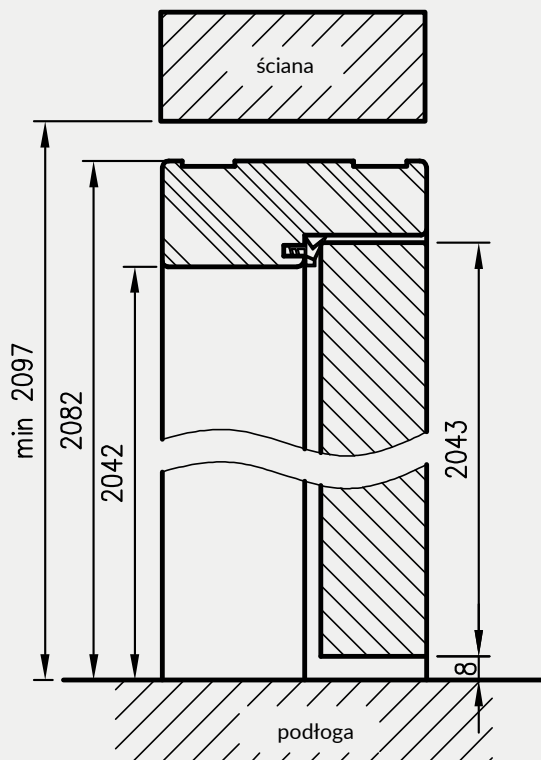
Przekrój pionowy OPB
