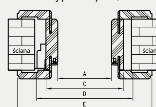
Przekrój poziomy OR/ORC
