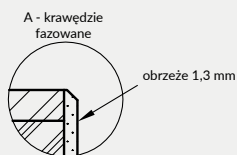
Przekrój ramiaka skrzydła bezprzylgowego
