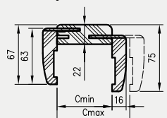
Przekrój TUN z ką. T80
