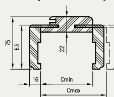
Przekrój OR/ORC z kąt. K63
