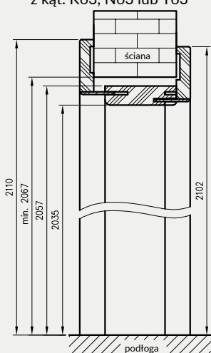
Przekrój pionowy tunelu regulowanego z ką. K63, N63 lub T63
