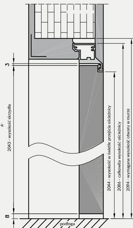
Profil ościeżnicy z uszczelką
