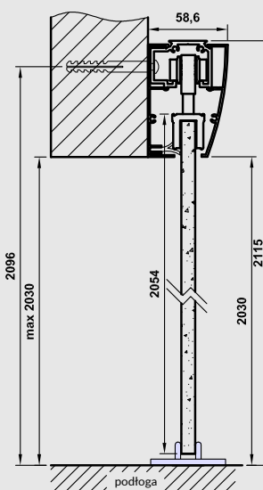
A - A przekrój pionowy systemu Spazio TO
