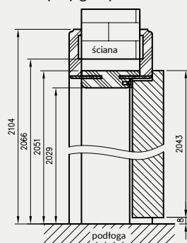
Przekrój pionowy drzwi przylgowych OR
