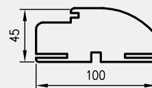
profil OP SOFT NATURA
