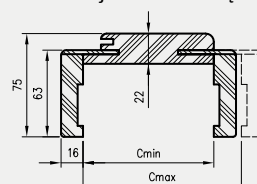
Przekrój OR/ORC z ką. T80
